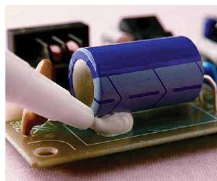
ФИКСАЦИЯ КРУПНОГАБАРИТНЫХ КОМПОНЕНТОВ НА ПЛАТЕ
