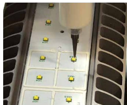
ГЕРМЕТИЗАЦИЯ СВЕТОТЕХНИЧЕСКОЙ ПРОДУКЦИИ И ФИКСАЦИЯ ВТОРИЧНОЙ ОПТИКИ
